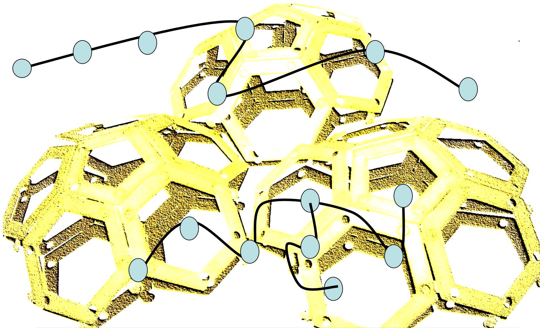
ESTRUCTURA DEL CLATRATO RODEADO DE MOLECULAS DE AGUA
